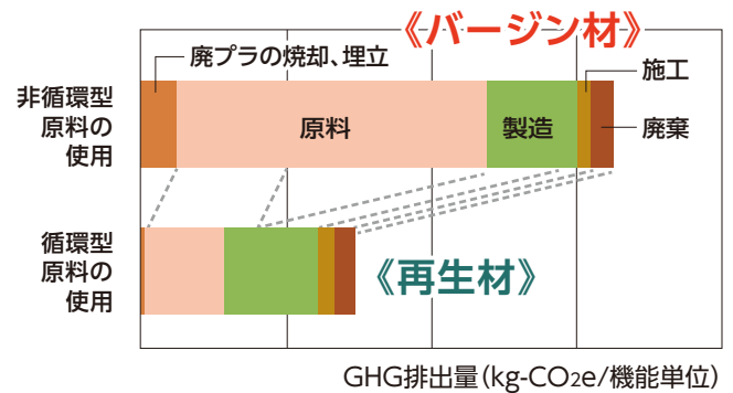
図19 循環型原料を使用した場合の 「気候変動」及び「資源の利用」にもたらされる効果
